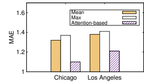
(b) MAE.
