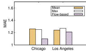
(b) MAE.
